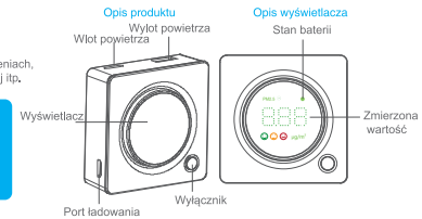
Czujnik PM2,5
